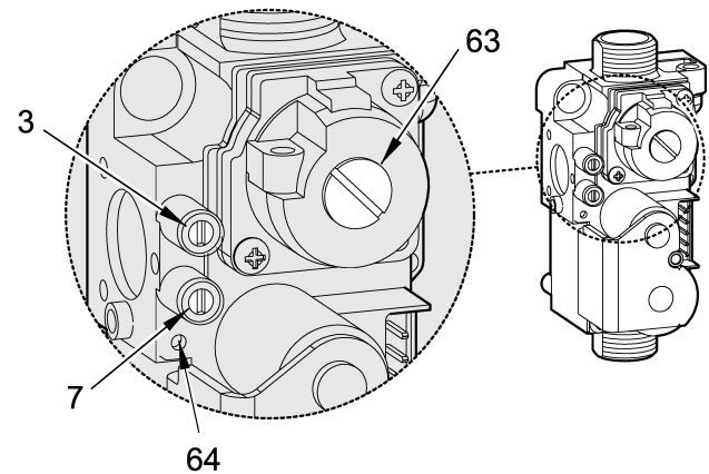
21 pav. Dujų armatūra.
